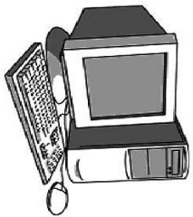
Hình 1.1: Máy tính
